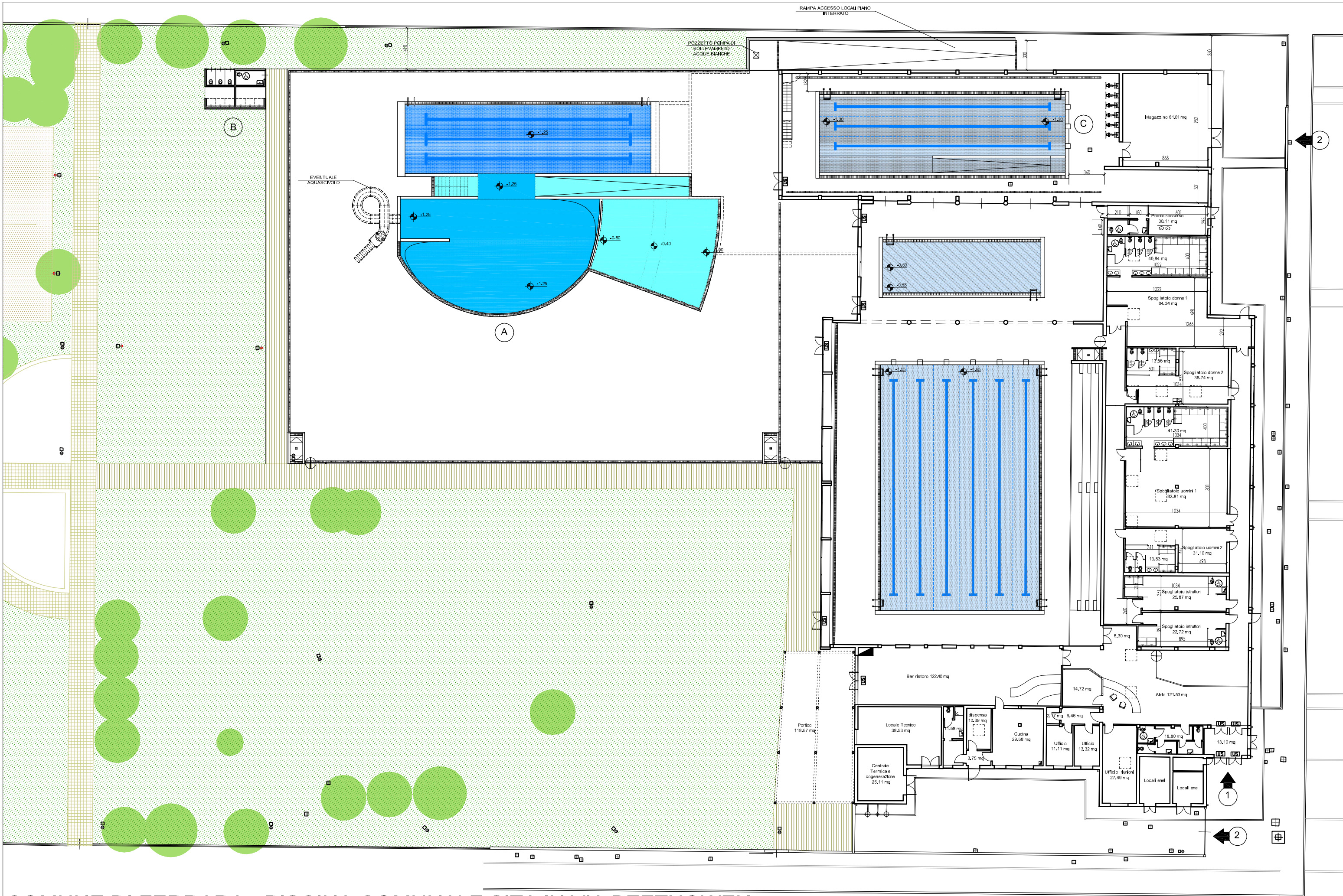
COMUNE DI FERRARA - PISCINA COMUNALE SITA IN VIA BEETHOVEN PLANIMETRIA PROGETTO PIANO TERRA
