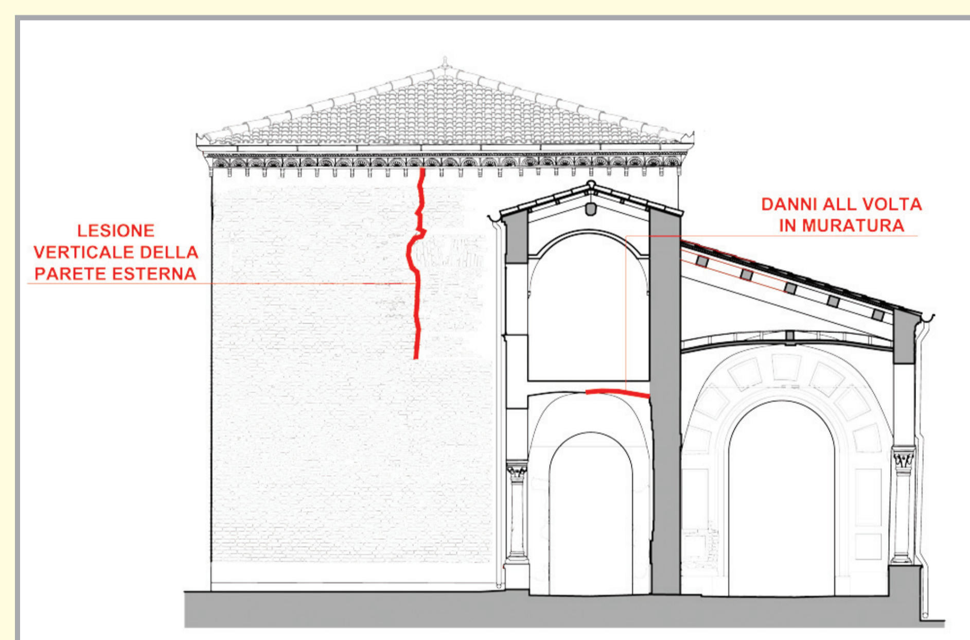
Cella Uomini Illustri nel Primo Gran Claostro Quadro fessurativo delle lesioni
