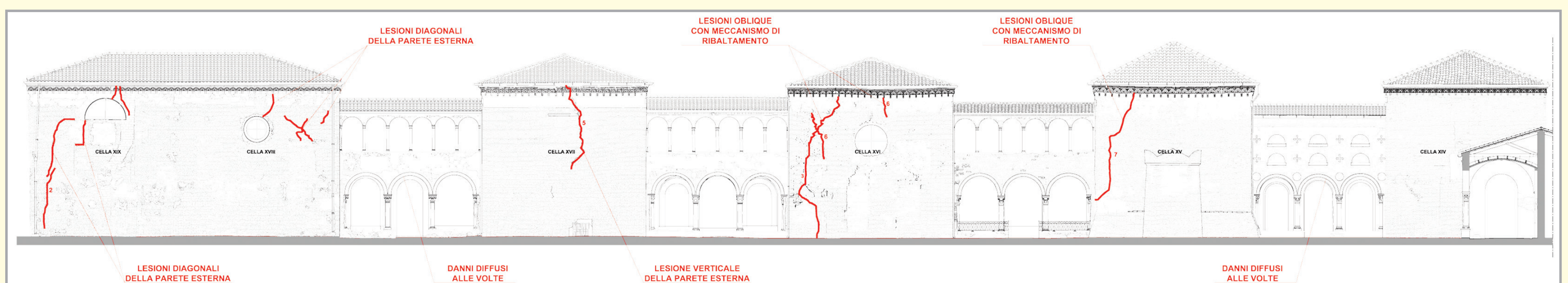
Primo Gran Claostro - Prospetto interno lato sud - Quadro fessurativo delle lesioni
