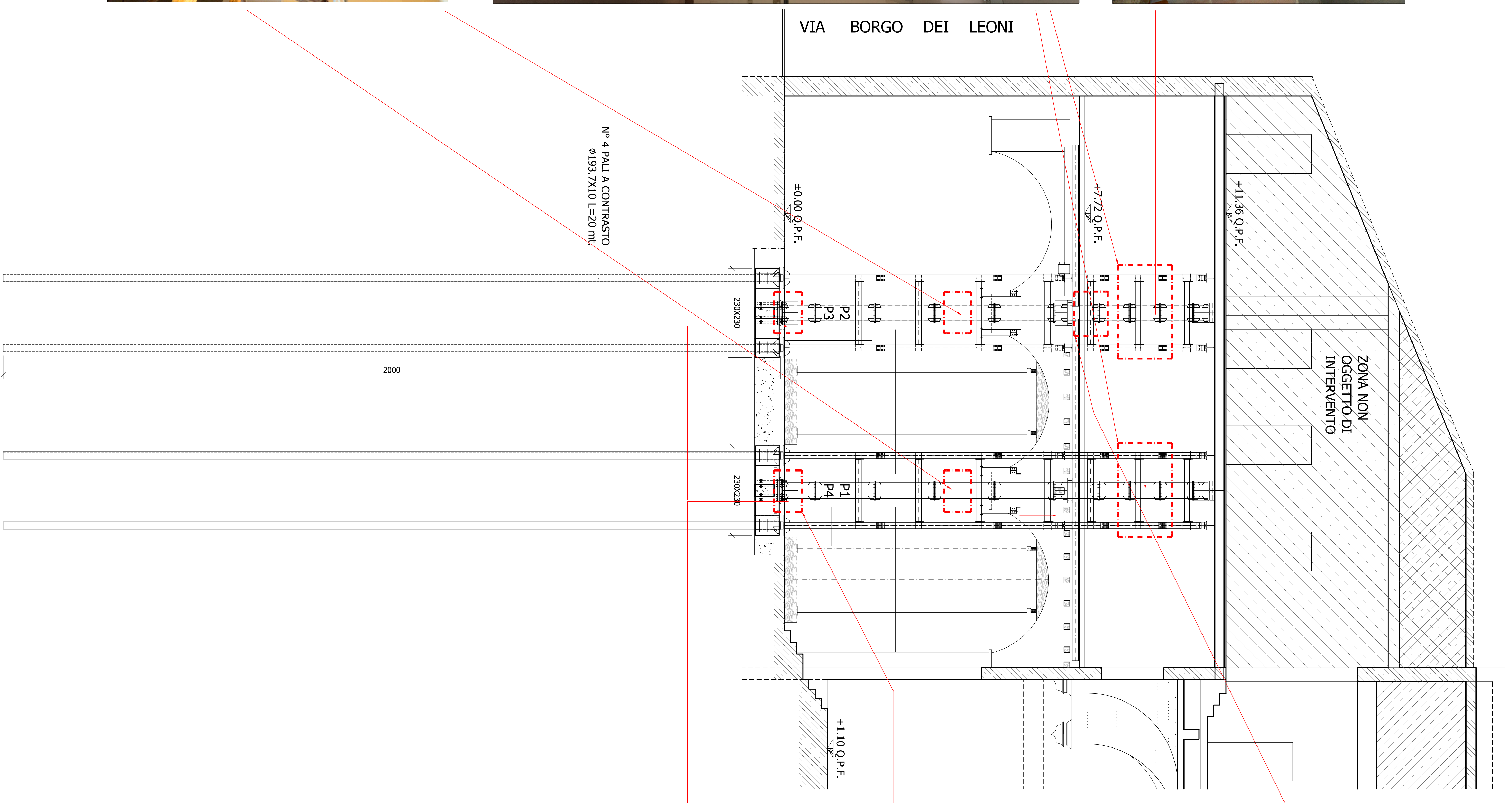
DETTAGLIO INTERVENTI DI RINFORZO DEI COLLEGAMENTI DELLE NUOVE COLONNE A LIVELLO DEL SOLAIO DI PIANO PRIMO
