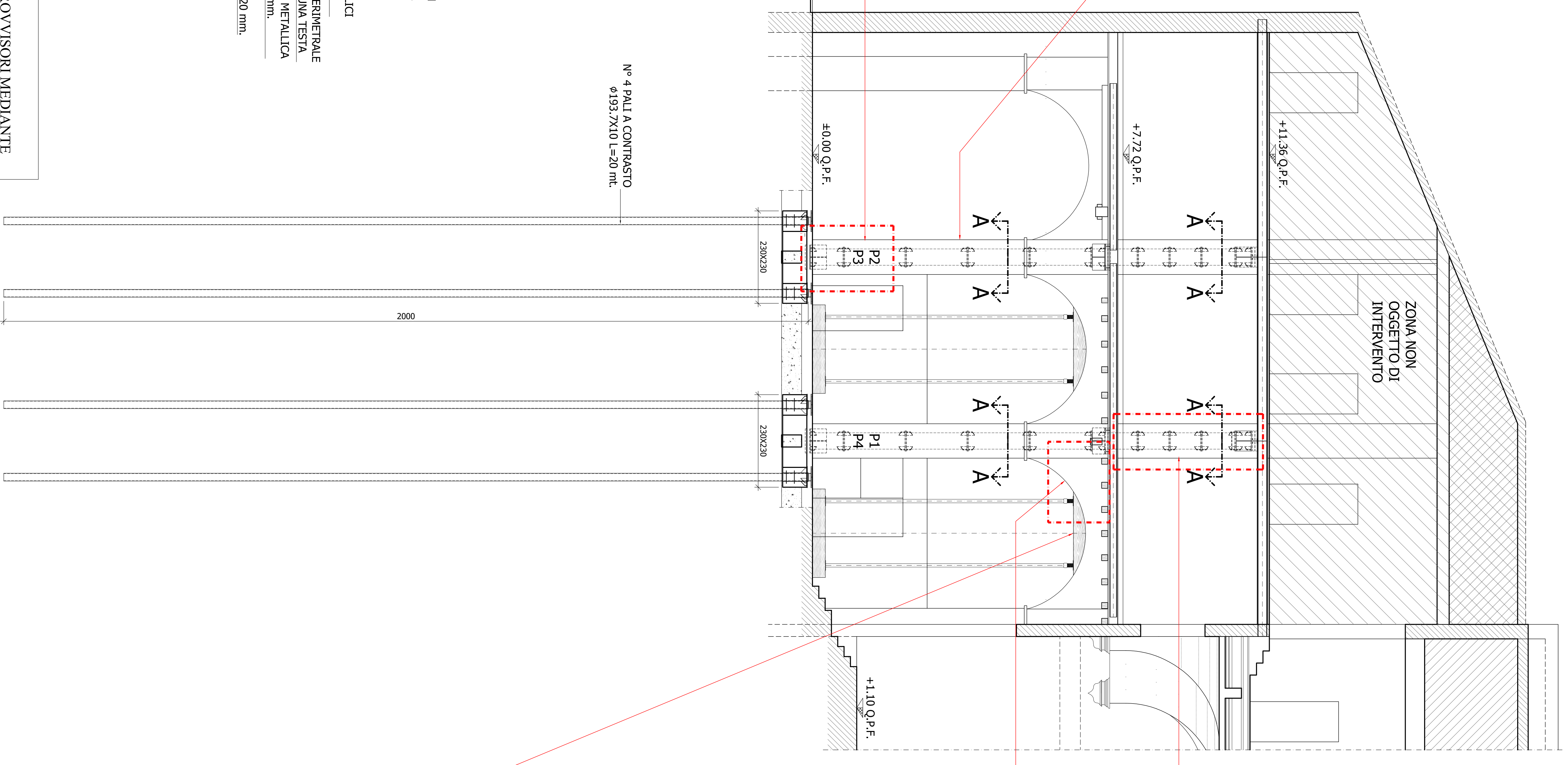
DETTAGLIO RICOSTRUZIONE FINALE RIVESTIMENTO IN MATTONI DELLE COLONNE METALLICHE
