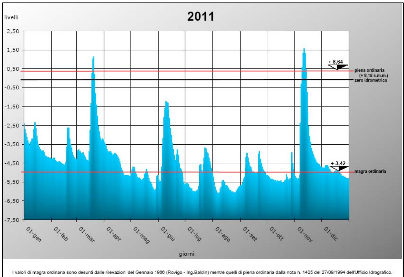
Graf. 1.39 - Livelli idrometrici giornalieri del fiume Po (m. rispetto allo zero idrometrico), rilevati alle ore 8.00 presso l'idrometro di Pontelagoscuro per l'anno 2011
